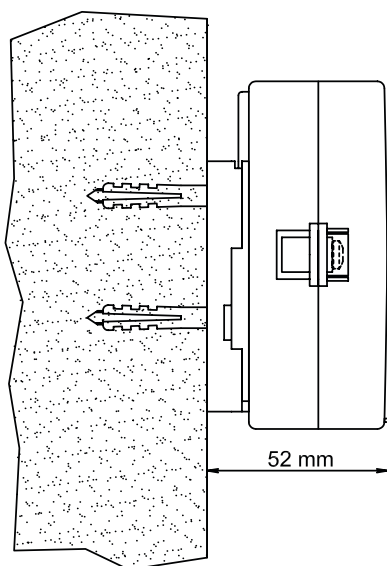
Montaż ścienny MULTICAL® 602 widok z boku
