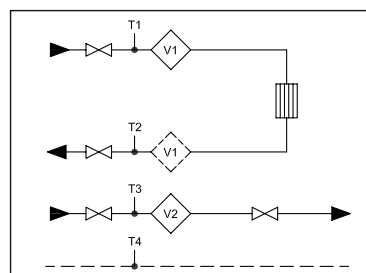
Przykład 2: System 2-przewodowy z 2 przetwornikami przepływu.
